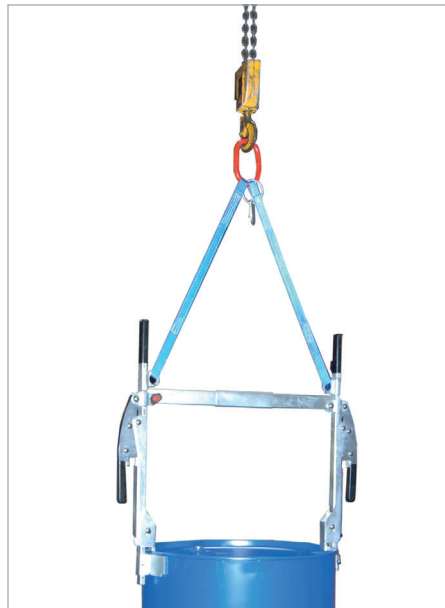
Aufnahme mittels Kran
